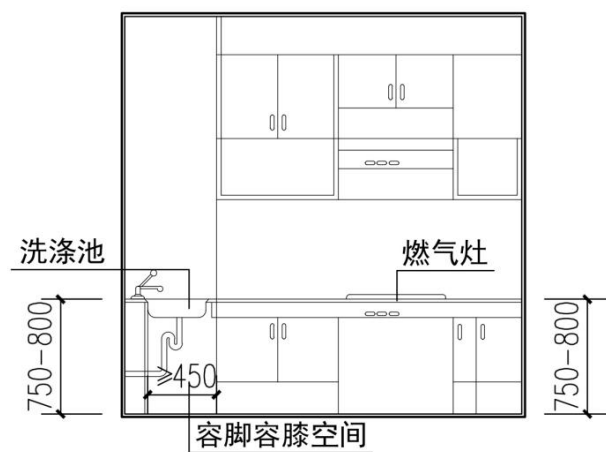
(b) 1-1 剖面图
