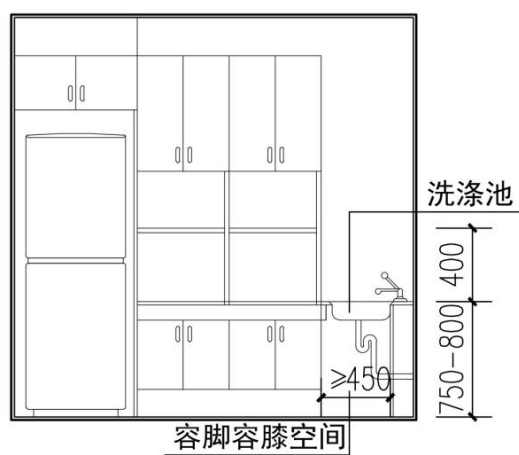
(b) 1-1 剖面图
