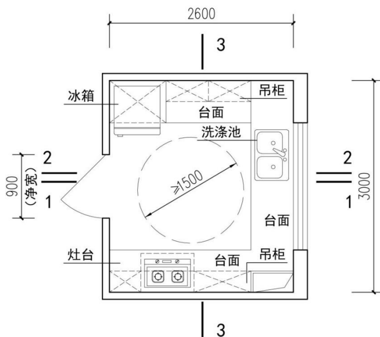
(a) 平面图
