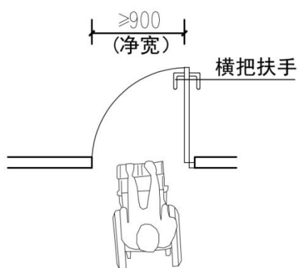
(g) 单扇平开门平面
